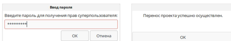
Рисунок 3.3 — Подтверждение импорта
