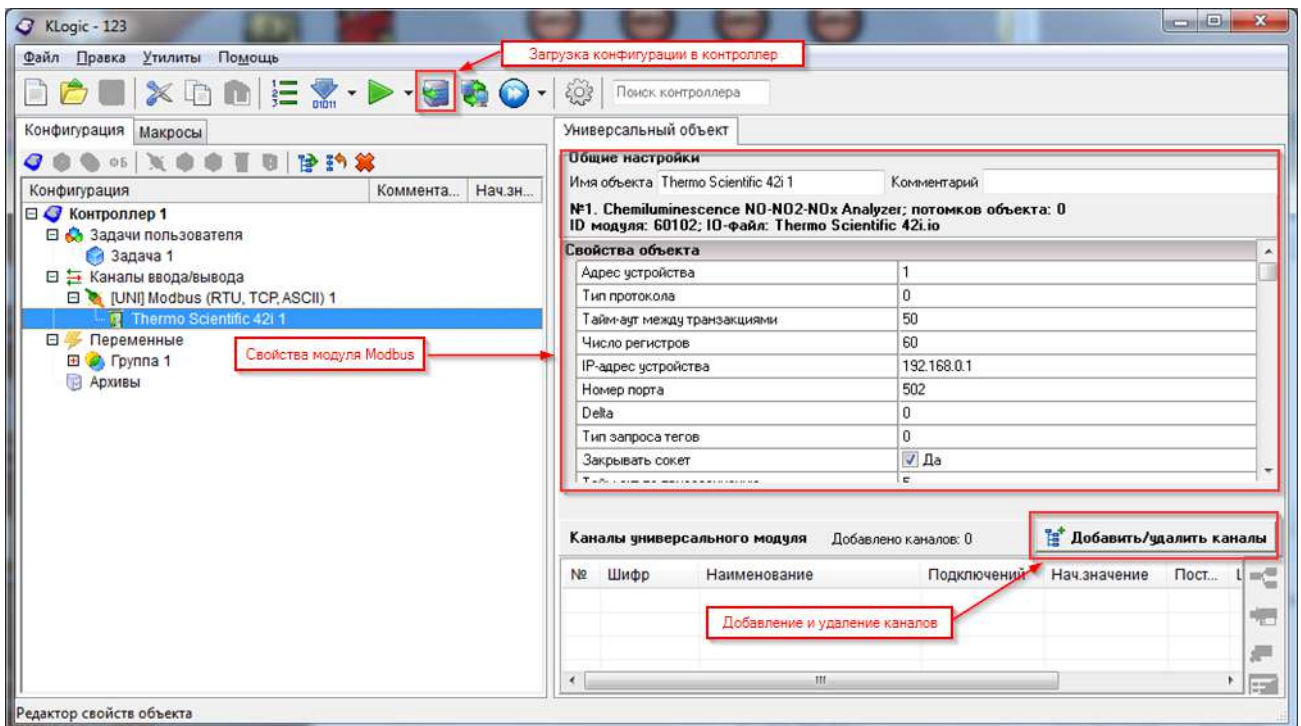
Рис. 9. Настройки устройства Modbus
